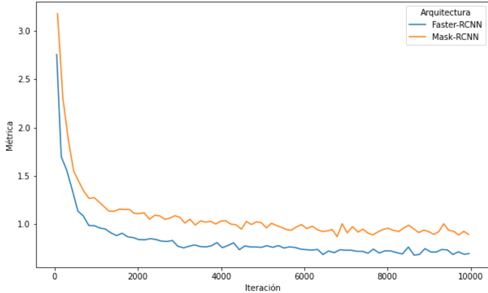
Figura 4.2: Desempeño según arquitectura de localización
