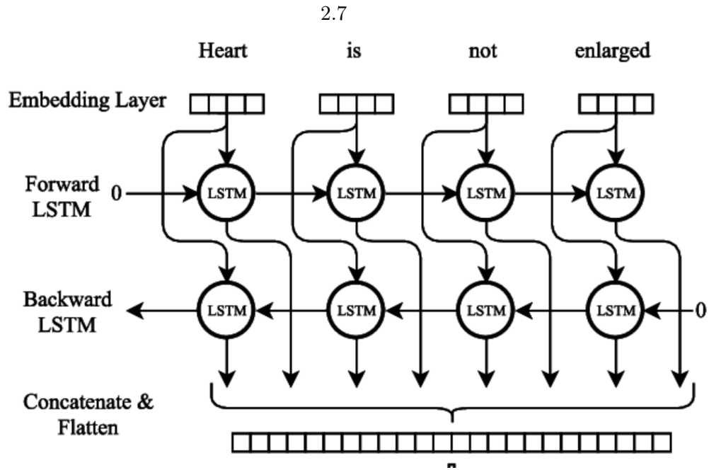
Figura 2.7: Arquitectura BiLSTM
