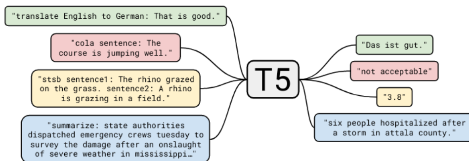
Figura 8: Diagrama de modelo unificado T5, tomado de [44]
