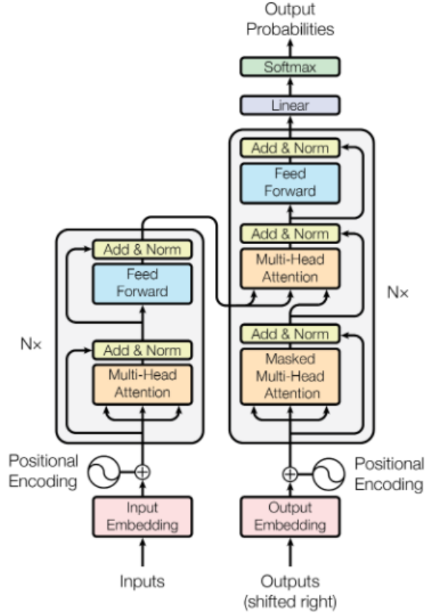
Figura 4: Transformers original, tomado de [55]
