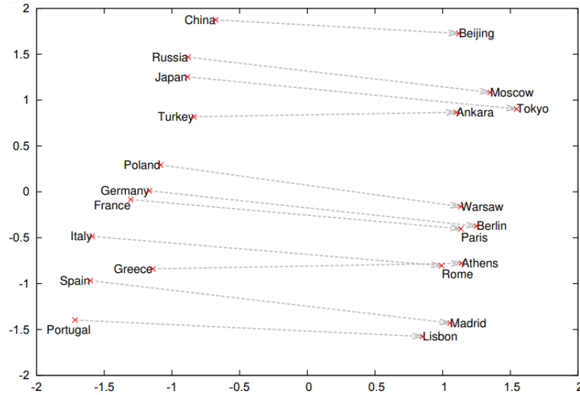
Figura 19: Vectores proyectados con PCA
