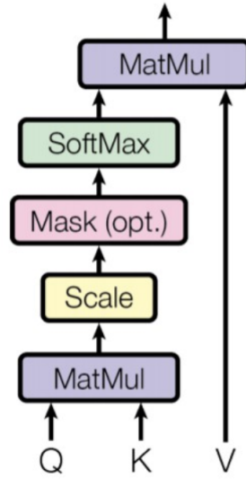
Figura 5: Mecanismo de atención, tomado de [55]
