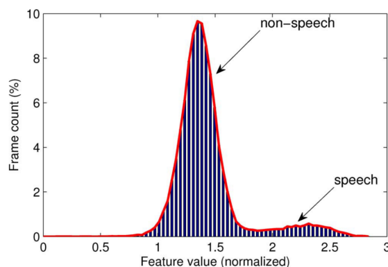
Figura 5: Distribución del descriptor combinado para una señal de audio arbitraria [17].
